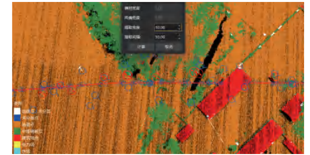
提取风偏点
